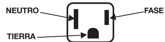
CONFIGURACIÓN DE RECEPTÁCULO NEMA 5-15R
